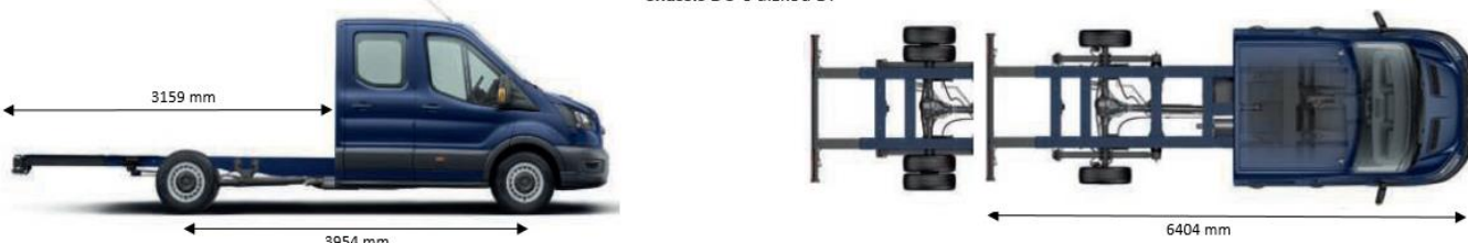
Chassis DC s dĺžkou L4
